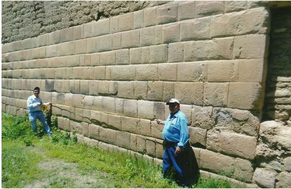
Realizando mediciones del muro norte de Huaytará en 2017.
